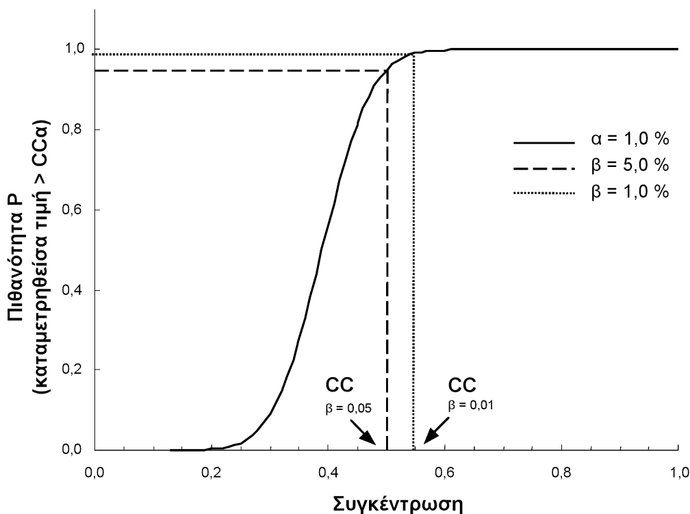
Σχήμα 1 Καμπύλη ισχύος
