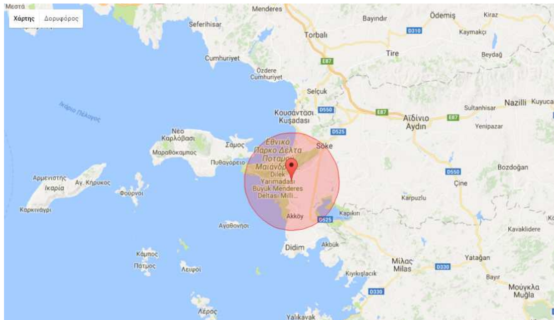
Εικόνα 1. Εστία και Ζώνη περίπου 20 χλμ.
